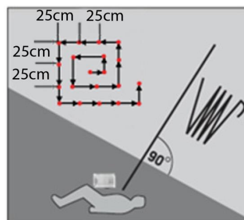
Shema spiralnega sondiranja. Razmak med spiralami in vbodi naj bo cca 25 cm.
